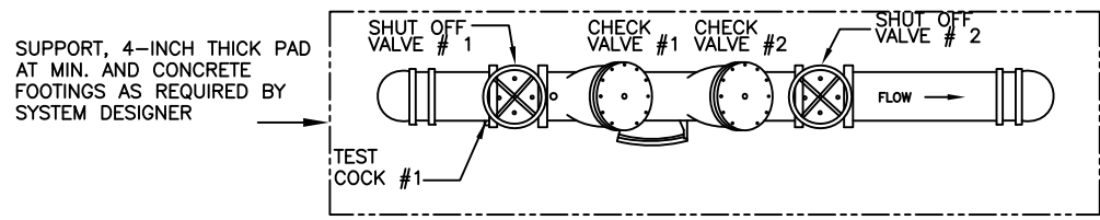
PLAN N.T.S.
